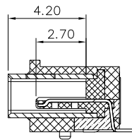
SEC: A-A
