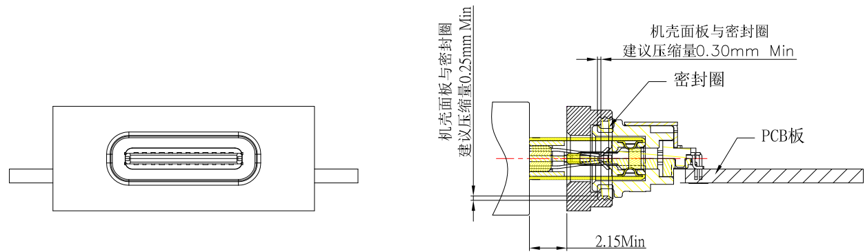
组装面板后公母头对插示意图
