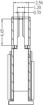
截面 2-2
