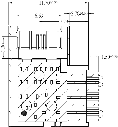
截面 3-3
