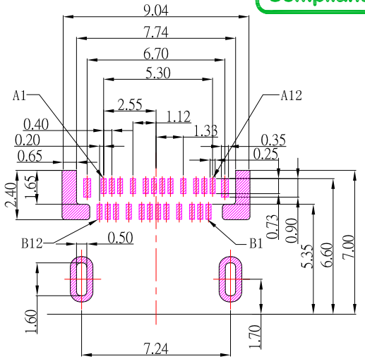
P.C.B LAYOUT
