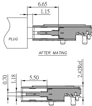
剖面图 比例1:1 A-A
