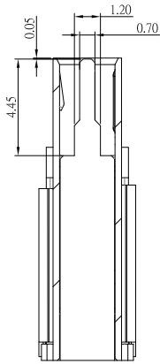
剖視圖
