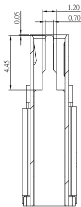
剖視圖
