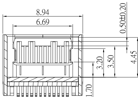
截面 1-1
