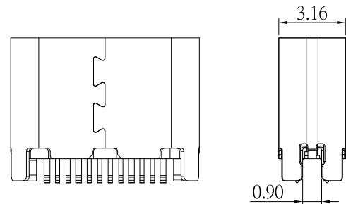
截面 A-A
