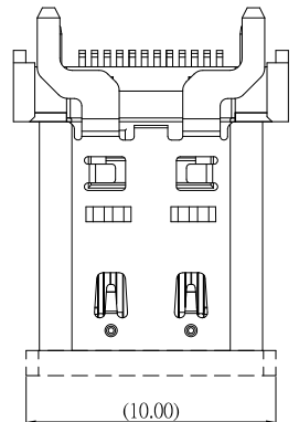
(COVER尺寸)
