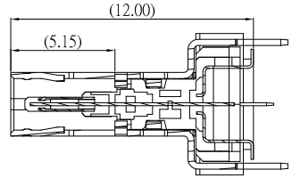
剖視"A-A" 比例 1:1
