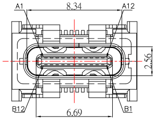
(COVER尺寸)
