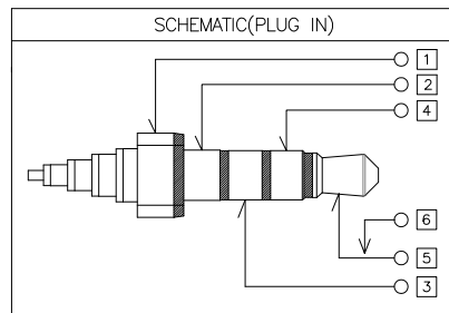
SCHEMATIC(PLUG IN)
