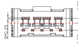
成品加CAP示意圖
