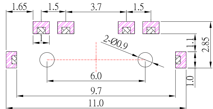
P.C.B LAYOUT
