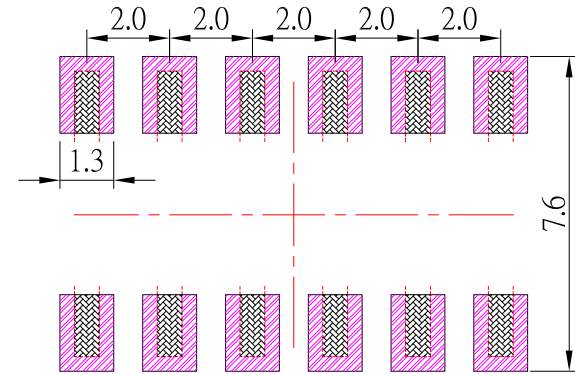
P.C.B LATOUT
