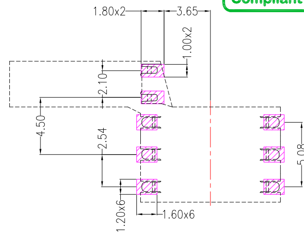
P.C.B Layout
