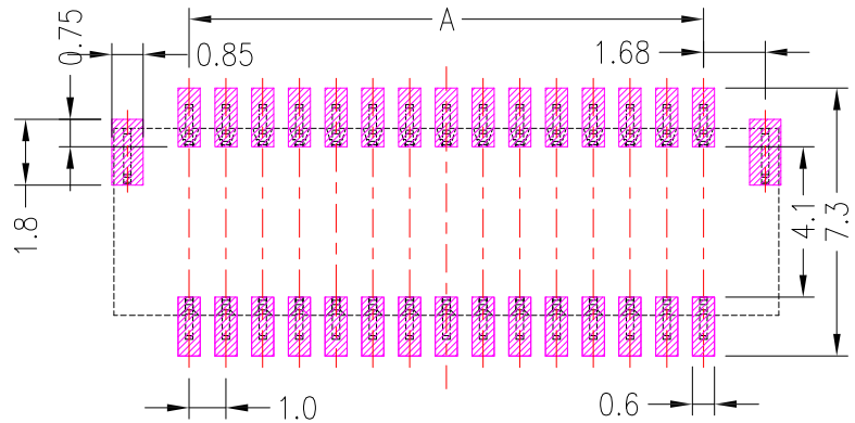
P.C.B LAYOUT
