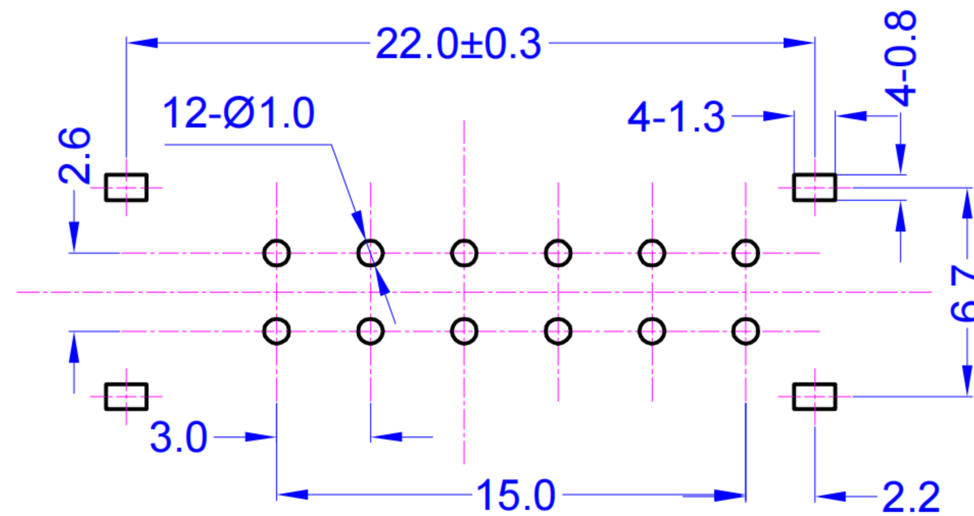
P.C.B LAYOUT
